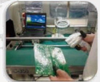
PCBA test
